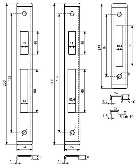
CE184/6U CE192V/6U CE296S/6U CE296S/10U
