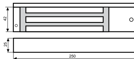
Model 13600M - wersja podstawowa Model 13700M - wersja z przełącznikiem NO/NC i sygnalizacją LED.
